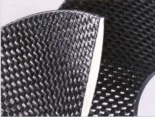
Nein, das sind keine Waffeln, das sind Stücke der Aerofoil-Bassmembran, die unterschiedlich dick gefertigt werden
